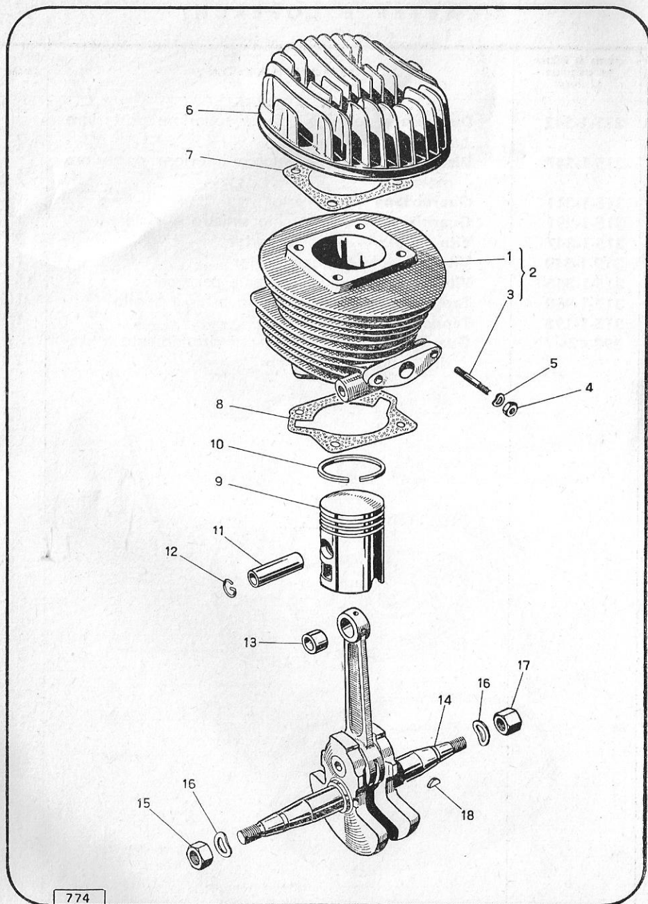
COMPLESSO 2 - CILINDRO - TESTA - ALBERO MOTORE
