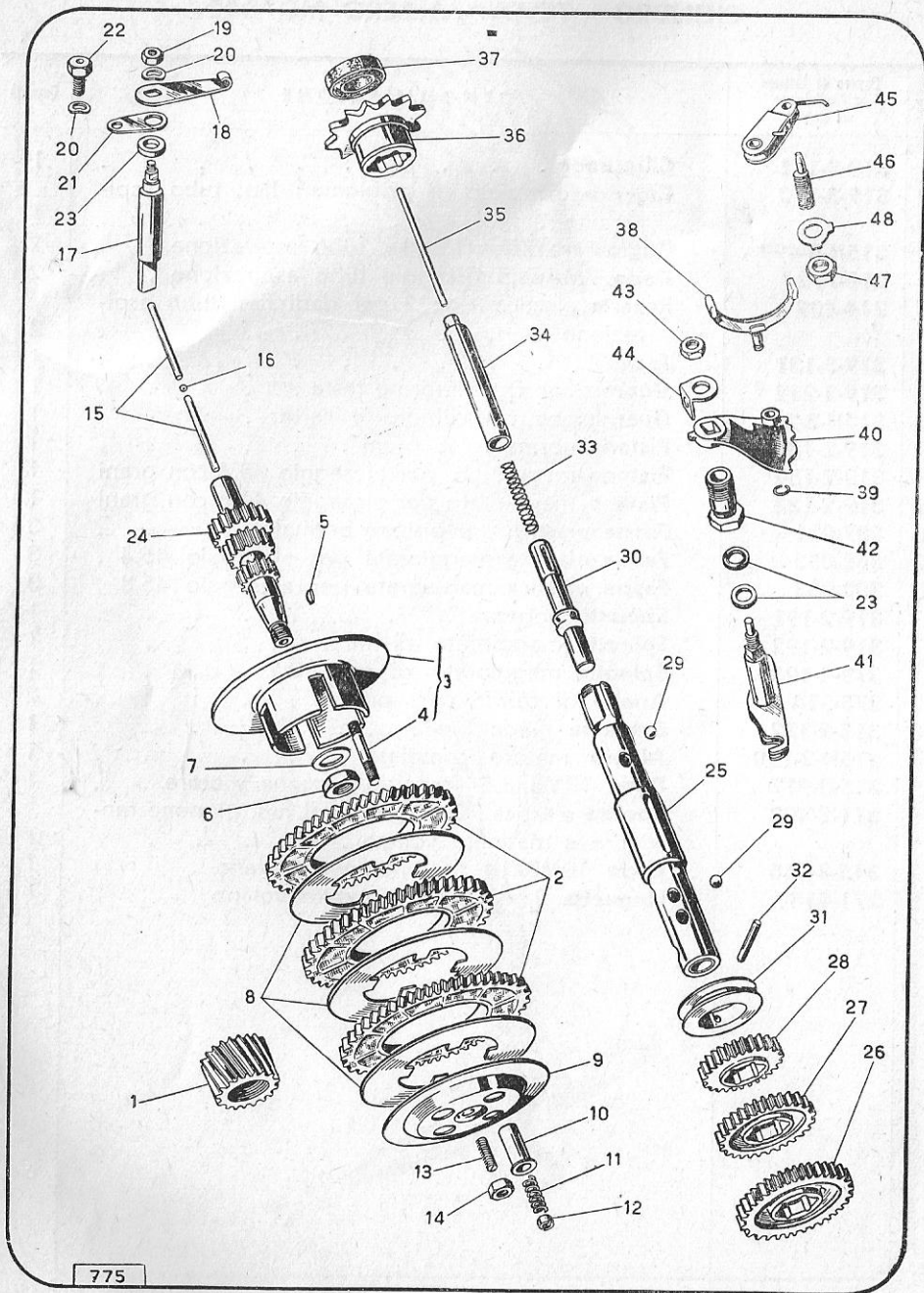
COMPLESSO 3 - FRIZIONE - CAMBIO DI VELOCITA'
