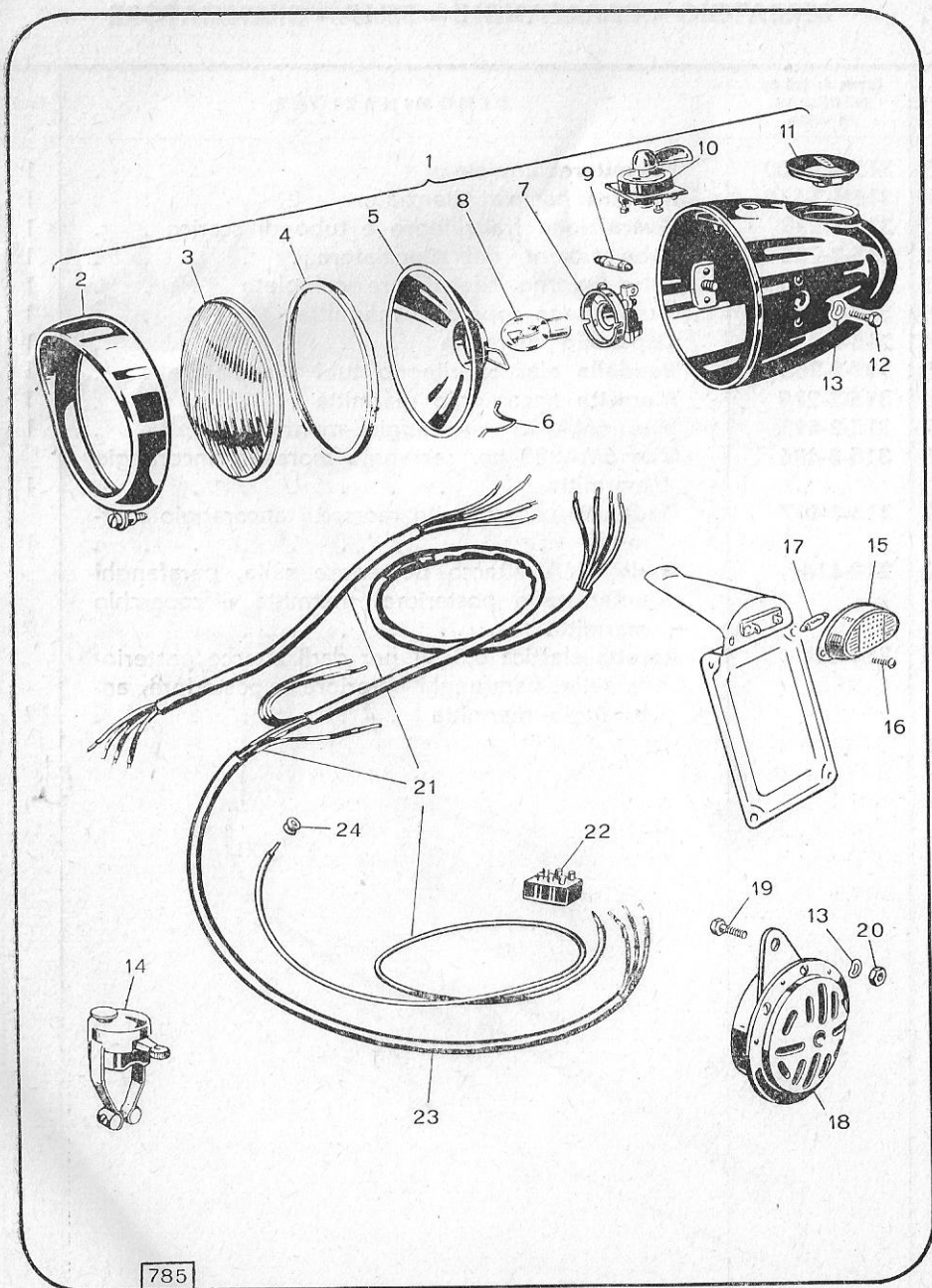
COMPLESSO 13 - IMPIANTO LUCE
