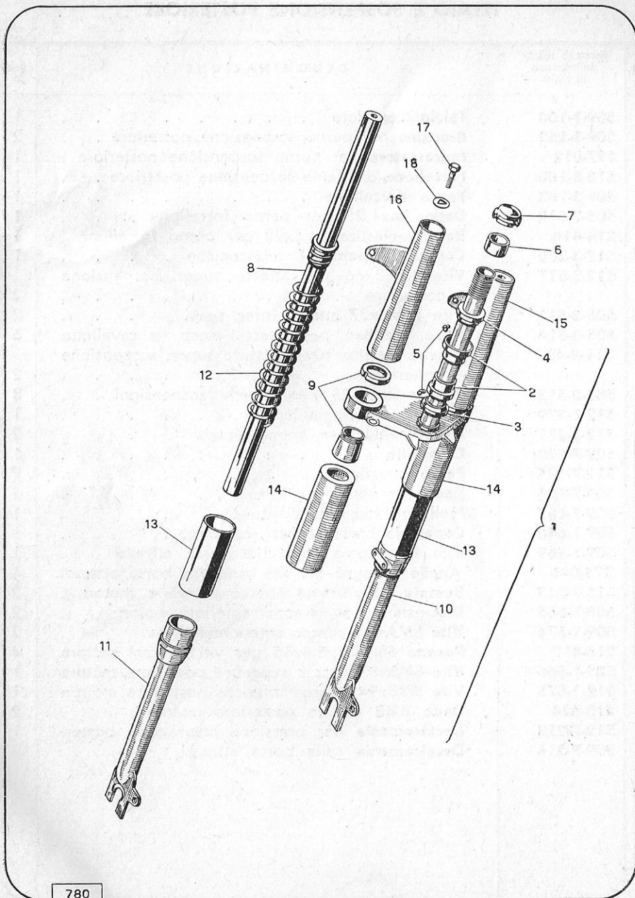
COMPLESSO 8 - FORCELLA TELESOPICA ANTERIORE
