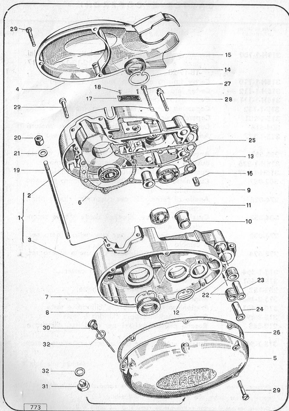
COMPLESSO 1 - CARTER E COPERCHI
