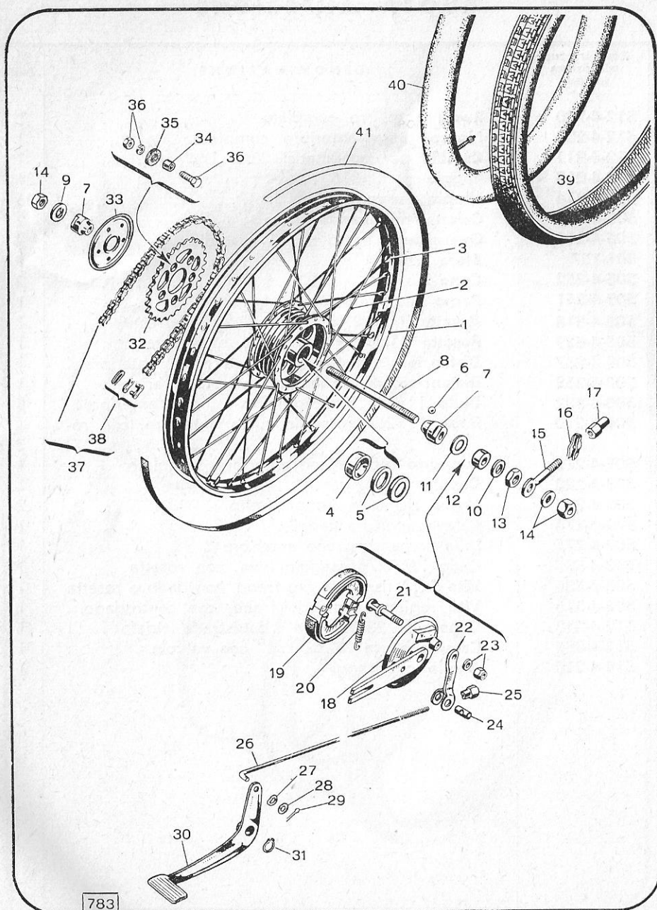
COMPLESSO 11 - RUOTA POSTERIORE
