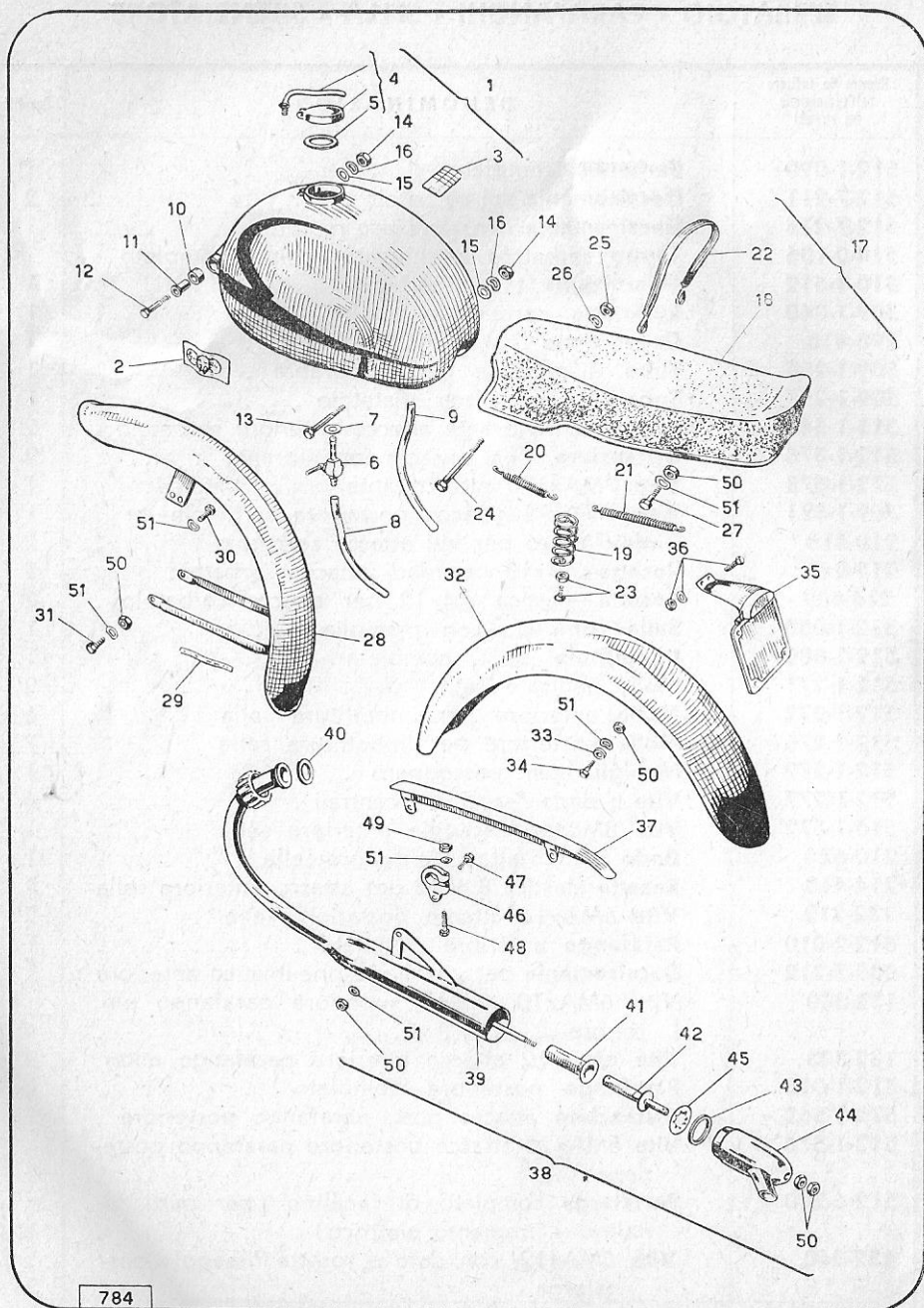
COMPLESSO 12 - SERBATOIO - PARAFANGHI - SELLA - SILENZIATORE
